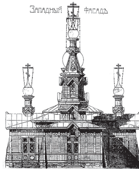
Церковь Иоанна Богослова, проект В.Н. Боброва
